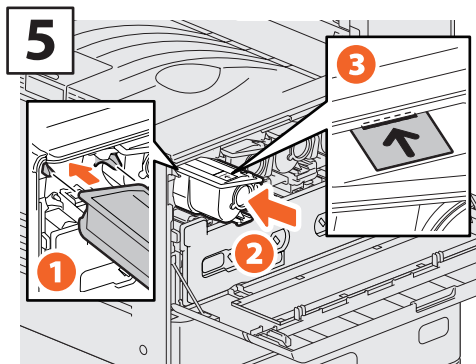
5 Wyrównaj nowy pojemnik z tonerem do prowadnic. Włóż go, aż do czarnej linii.
